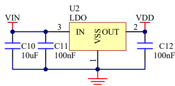
建议电源用LDO
