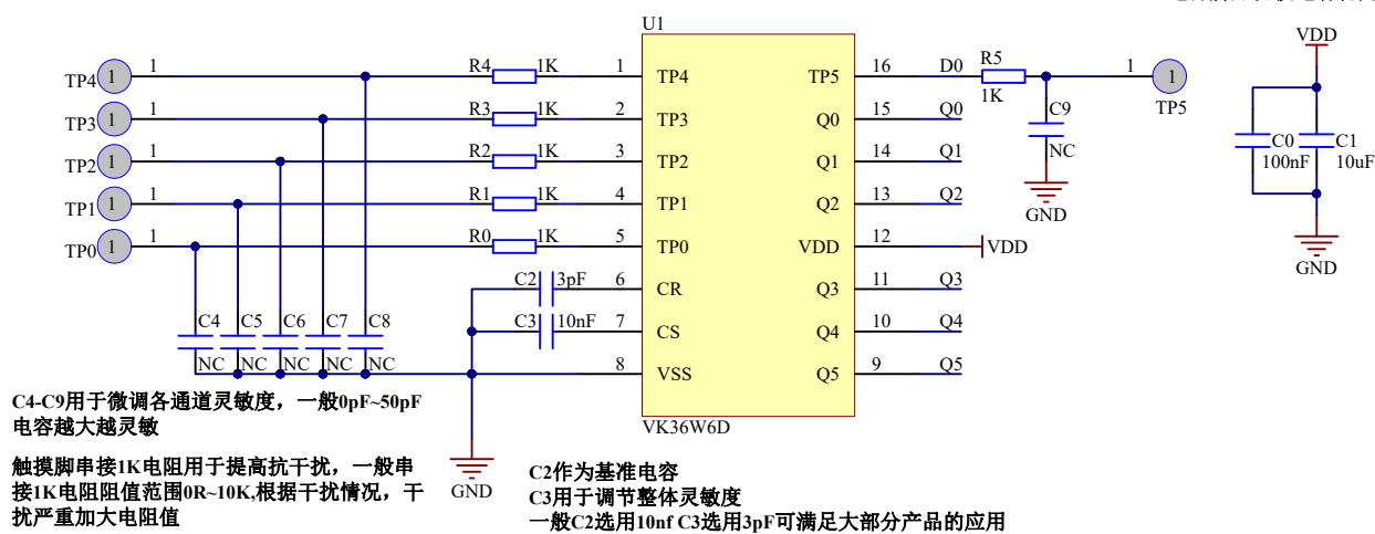
电源脚加滤波电容稳定电源
