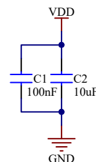
电源脚加滤波电容稳定电源
