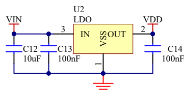
建议电源用LDO
