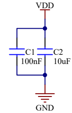
电源脚加滤波电容稳定电源
