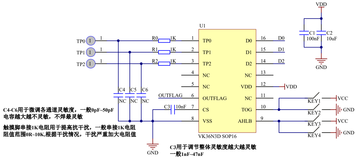
电源脚加滤波电容稳定电源
