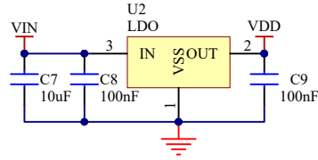
建议电源用LDO
